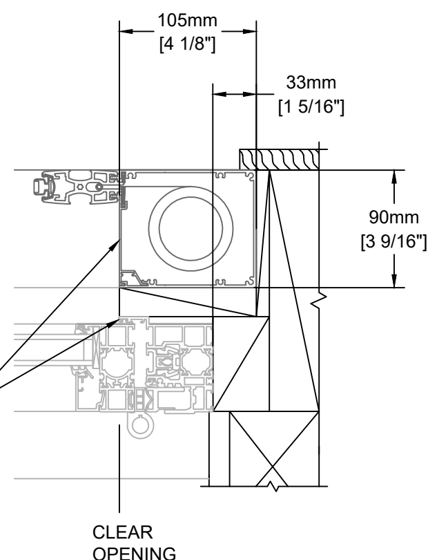
Horizontal Section Jamb Pivot
