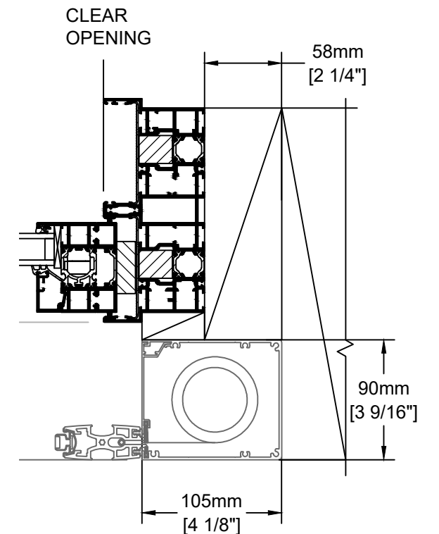
Horizontal Section Jamb Pivot
