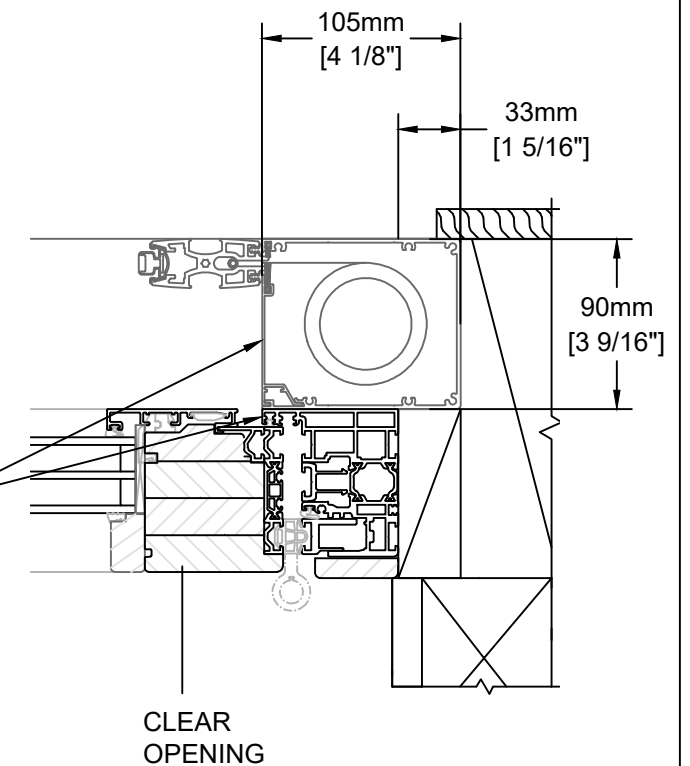
Horizontal Section Jamb Pivot
